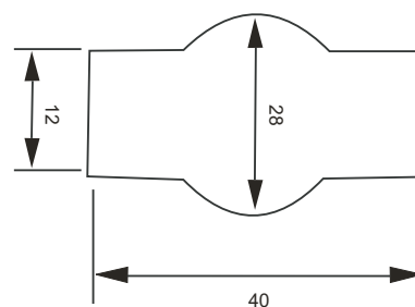
Bus Bar Dimension (mm) : 12 x 40, Ø28
